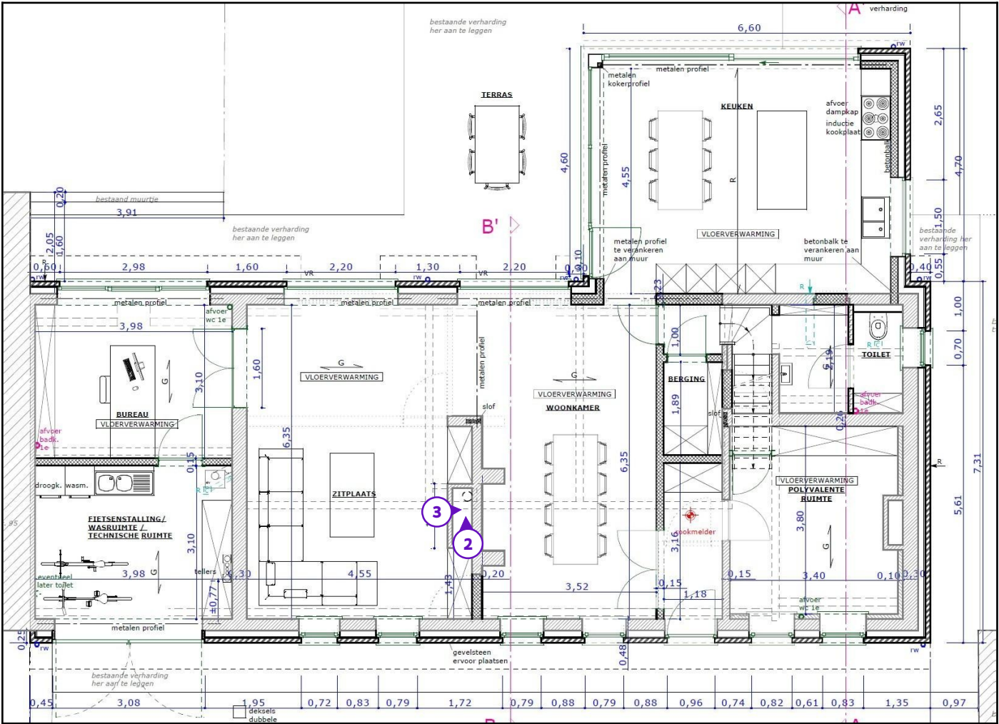
Legende van plan 1.1: Plan gelijkvloers
